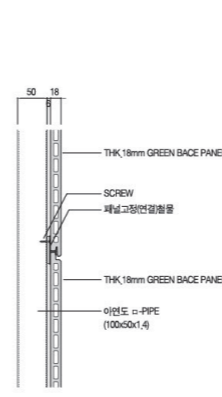
패널 연결부 단면 상세도
