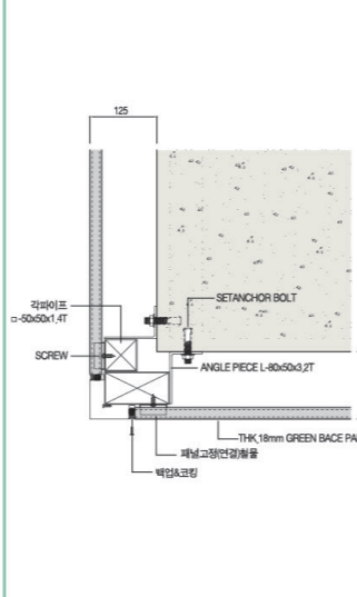
콘크리트구조 - 코너부위 상세도
