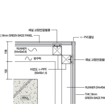
아웃코너 부분 상세도
