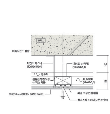
패널 후면부 골조보강(응벽고정)평면상세도
