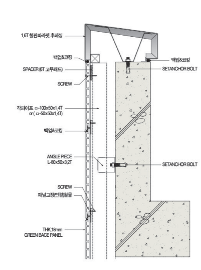
파라펫부위 상세도
