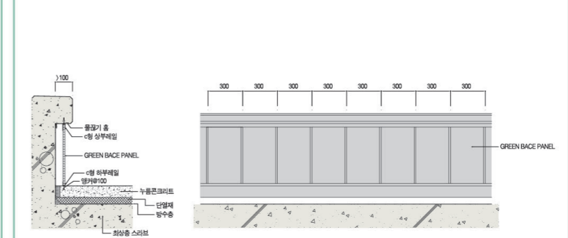
옥상 파라펫 상세도
