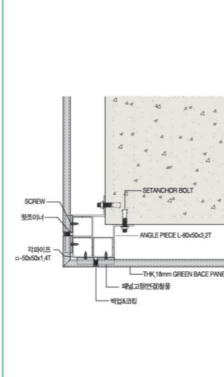
상단부 단면 상세도
